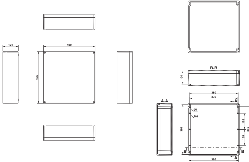
Disegno quotato
