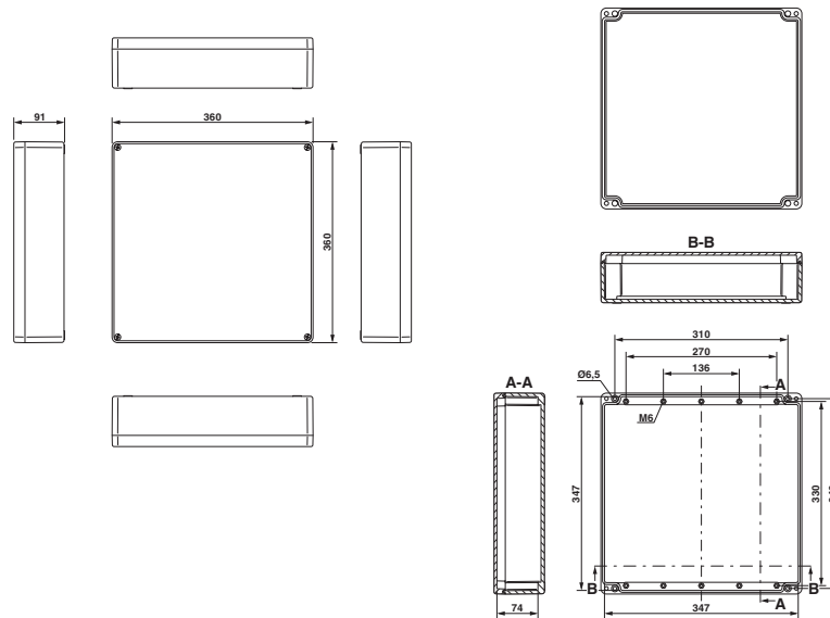
Disegno quotato
