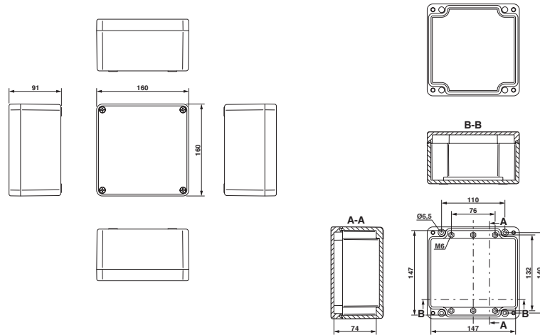
Disegno quotato
