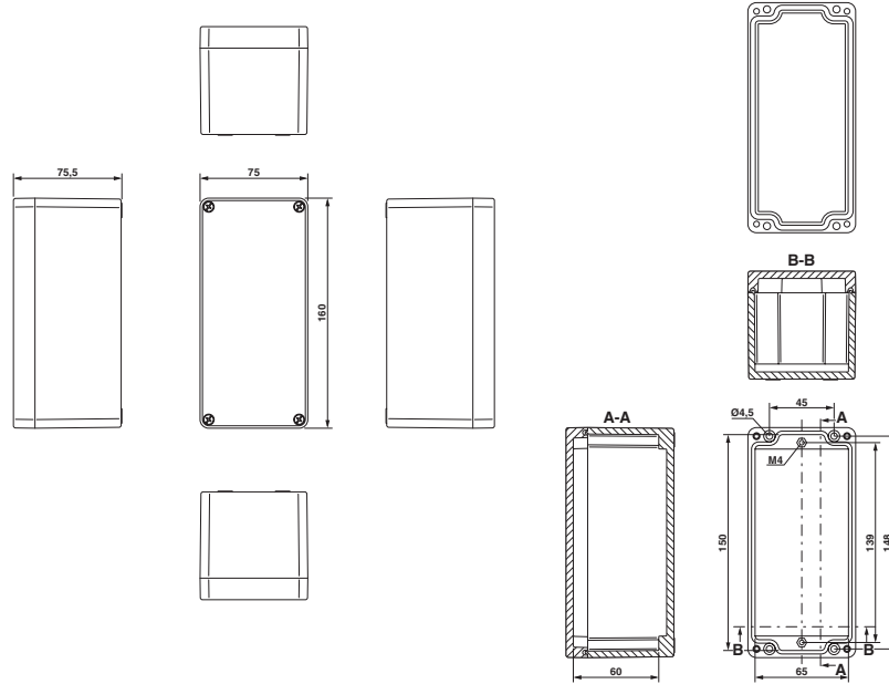
Disegno schema
