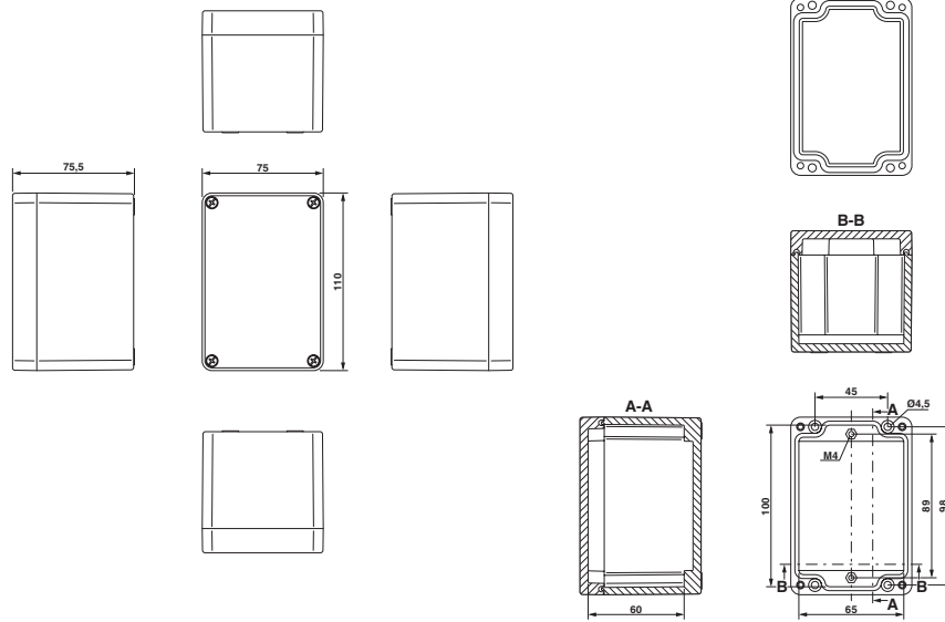
Disegno quotato
