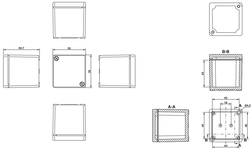
Disegno schema
