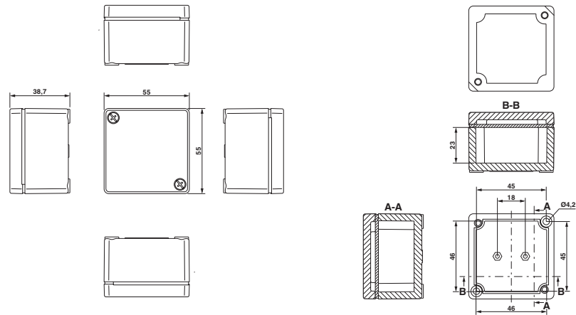
Disegno quotato
