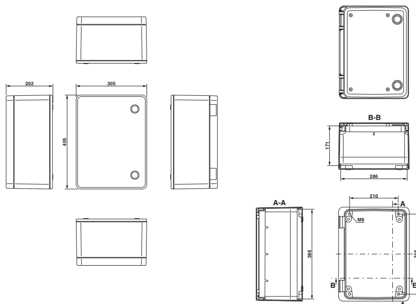
Disegno quotato
