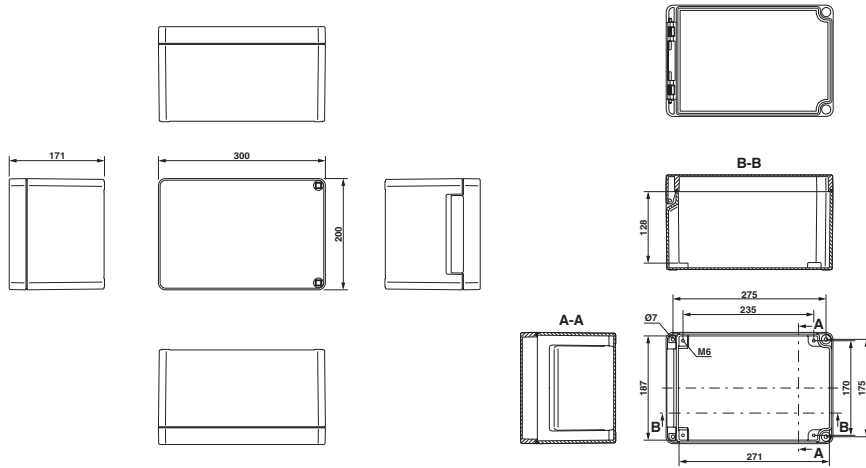
Disegno quotato
