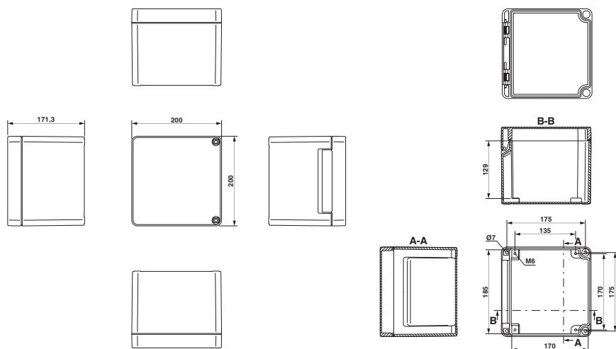
Disegno quotato
