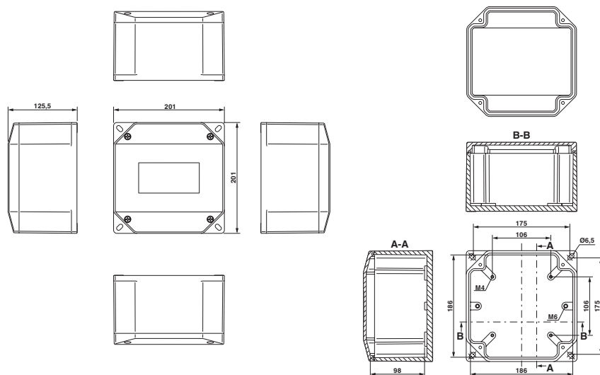
Disegno quotato
