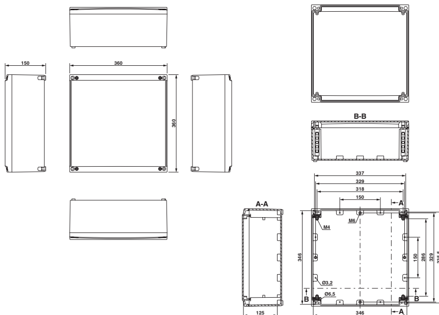
Disegno quotato
