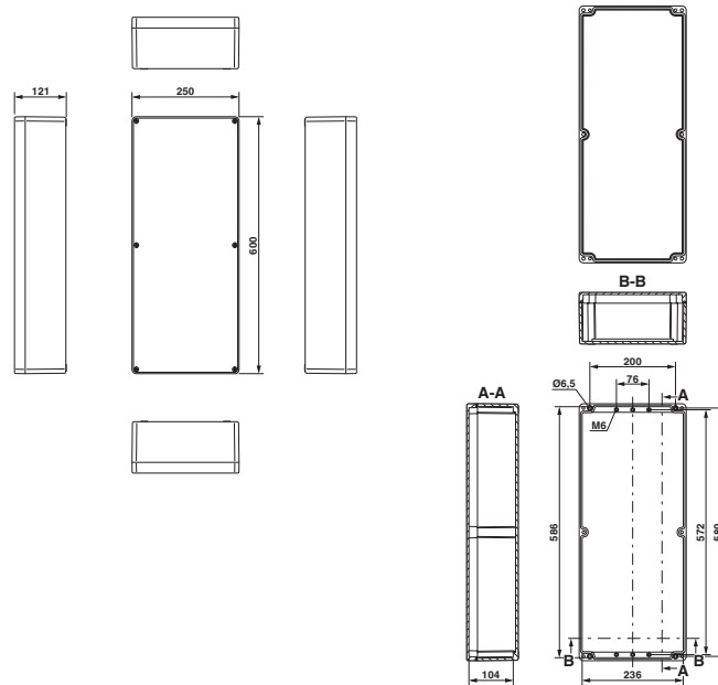
Disegno quotato
