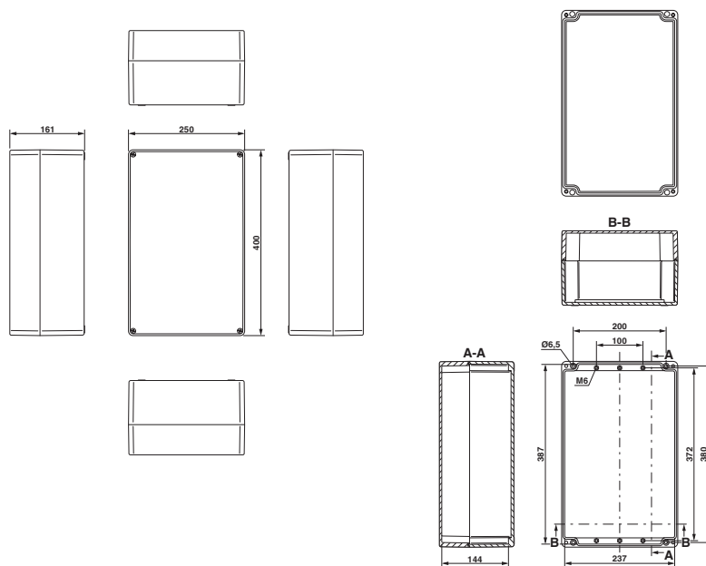
Disegno quotato
