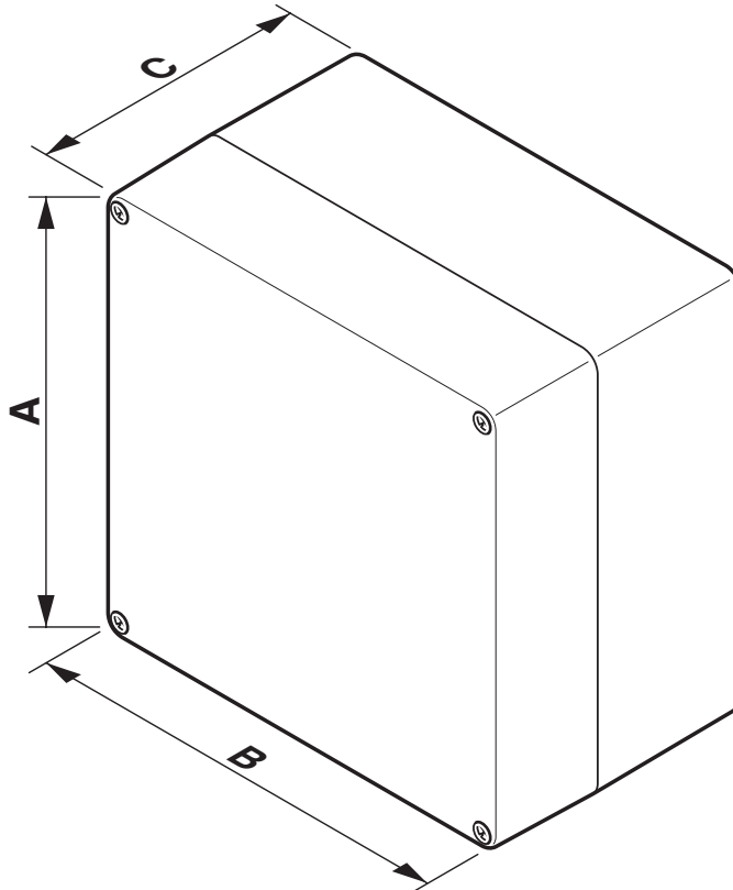
Disegno schema
