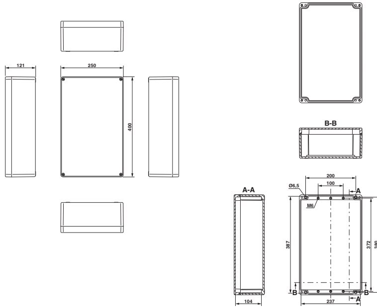
Disegno quotato
