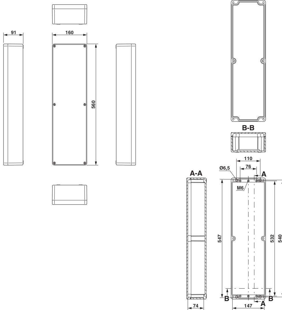
Disegno quotato
