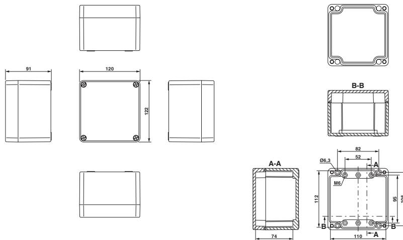
Disegno quotato
