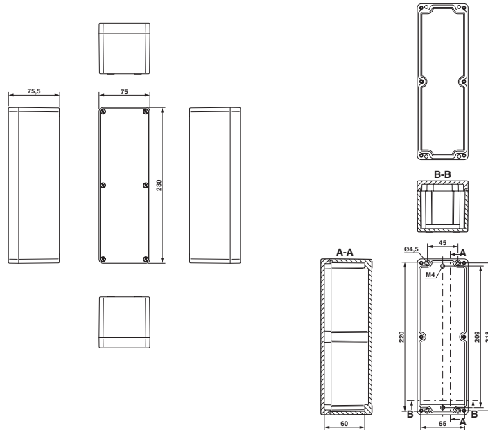
Disegno quotato
