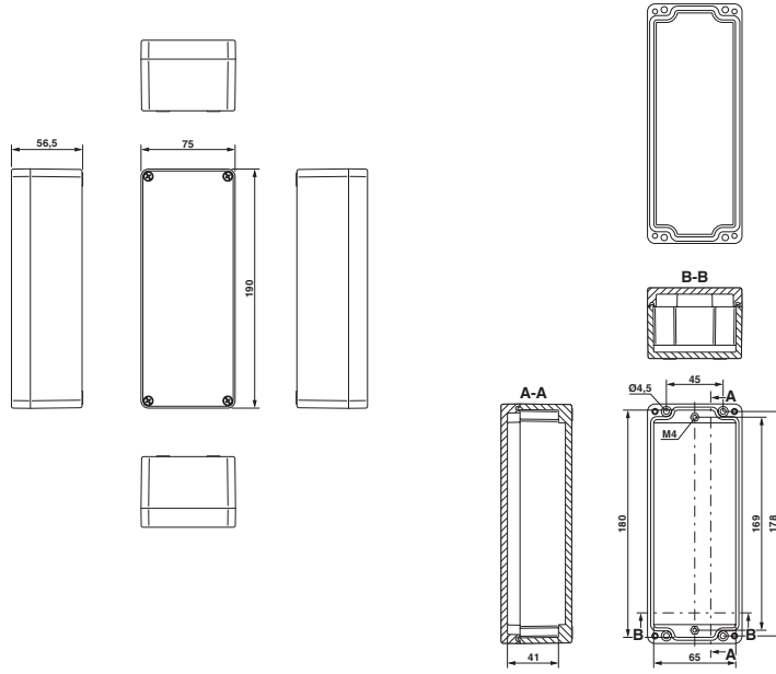
Disegno schema
