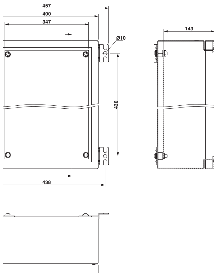
Disegno quotato
