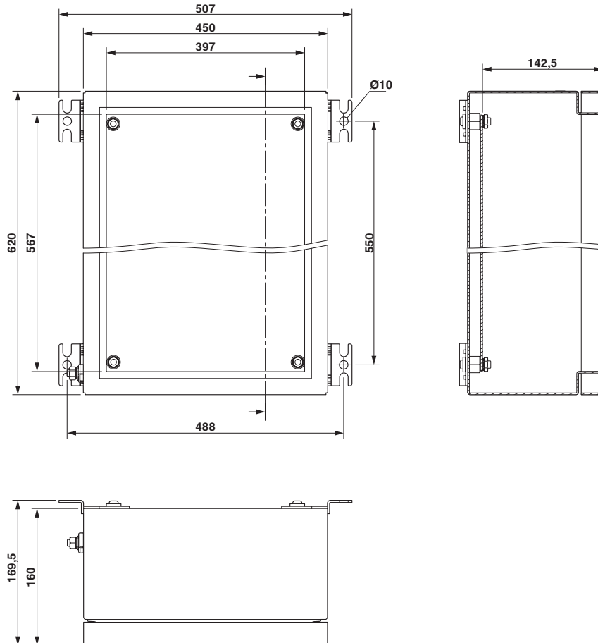
Disegno quotato
