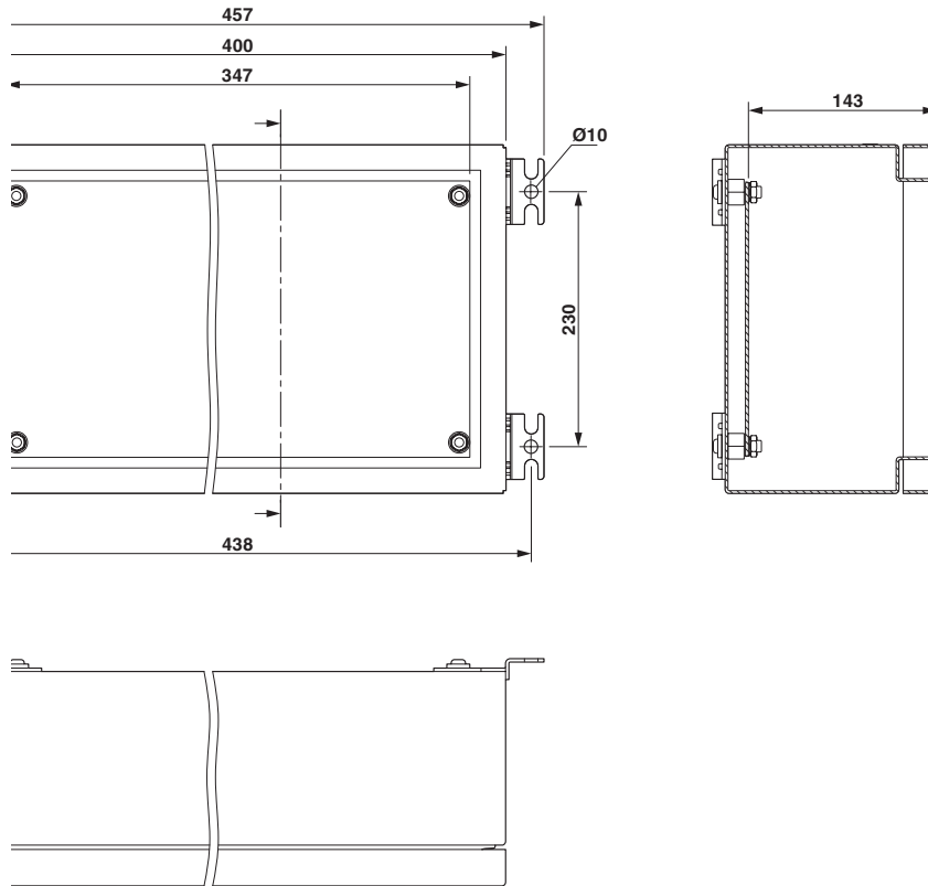
Disegno quotato
