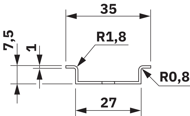
Disegno quotato
