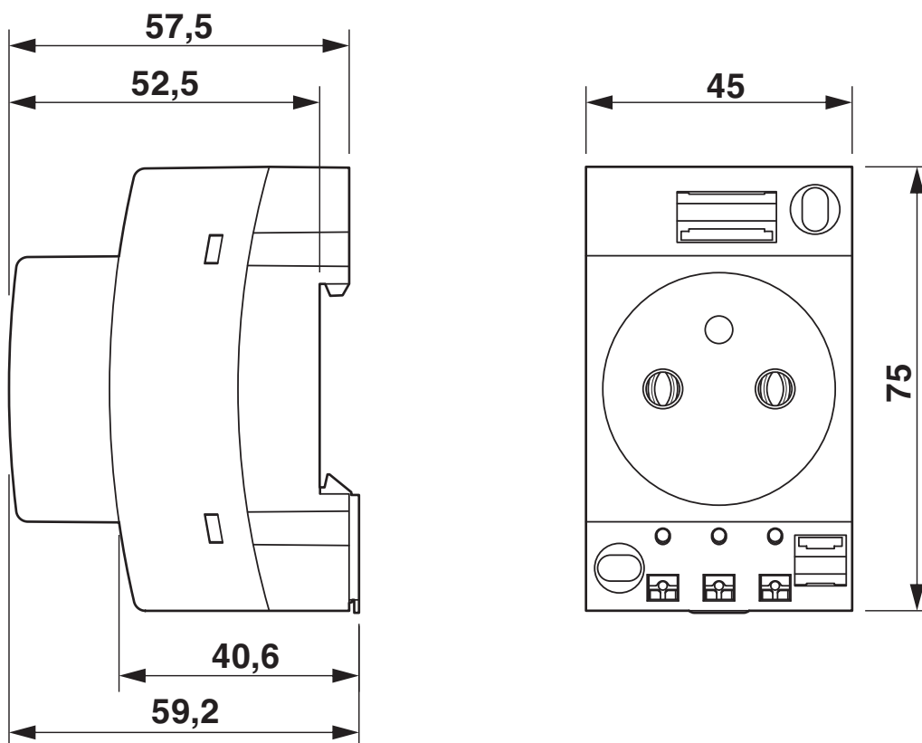
Disegno quotato
