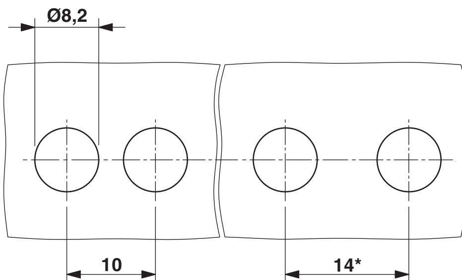
Disegno quotato
