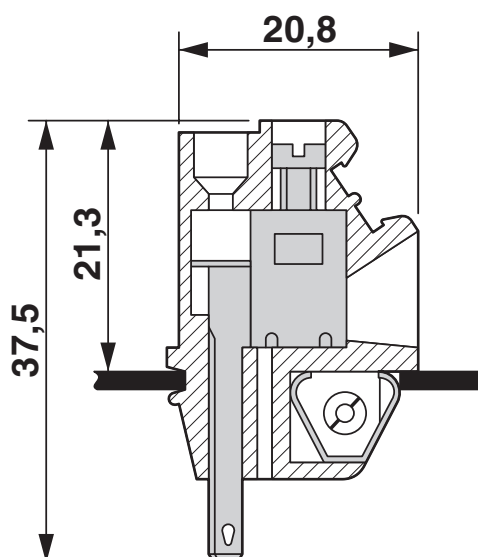
Disegno quotato
