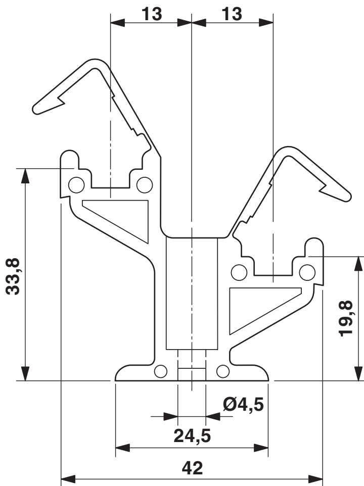
Disegno quotato
