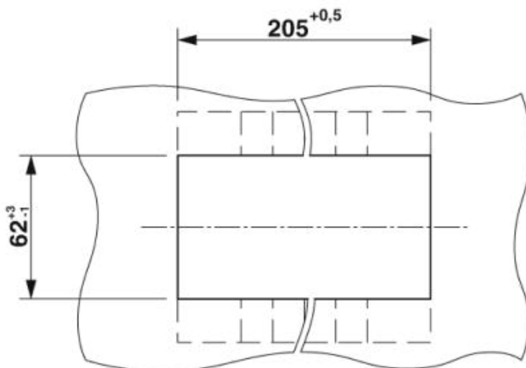
Disegno quotato
