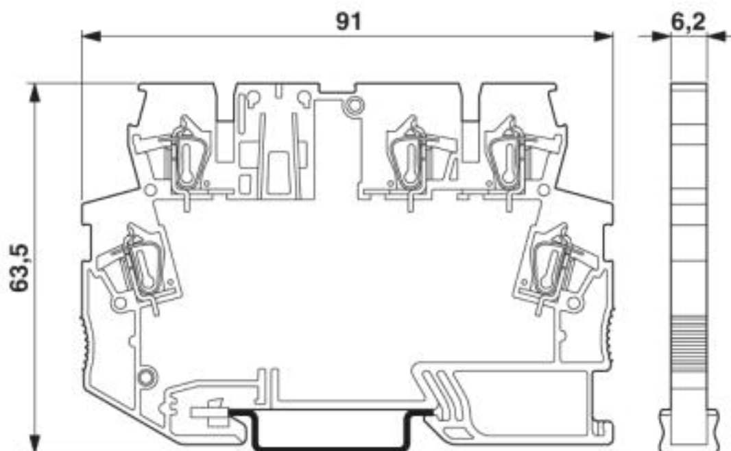
Disegno quotato
