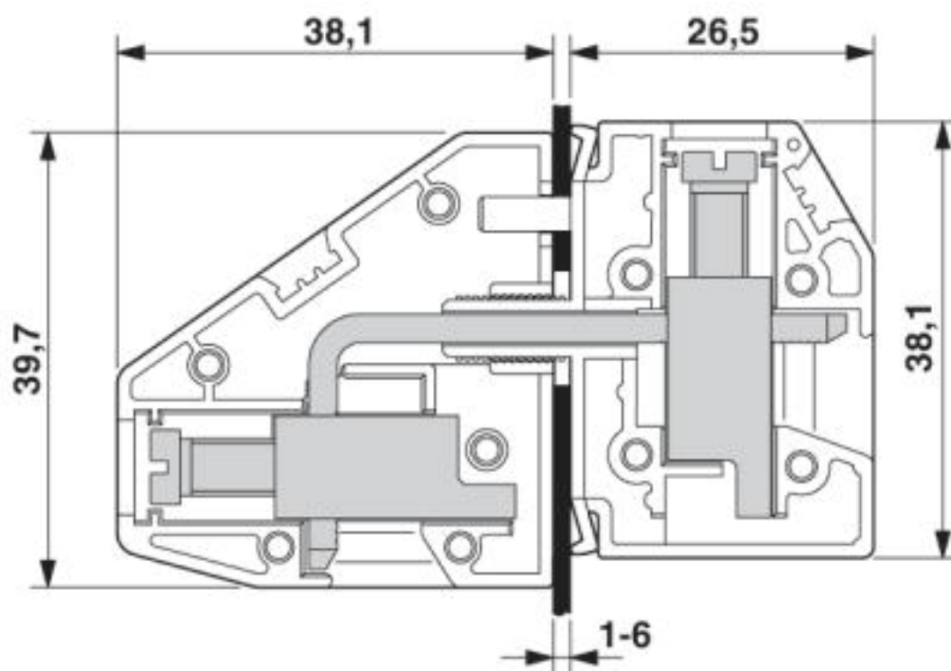
Disegno quotato
