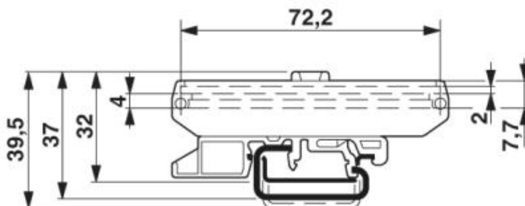
Disegno quotato
