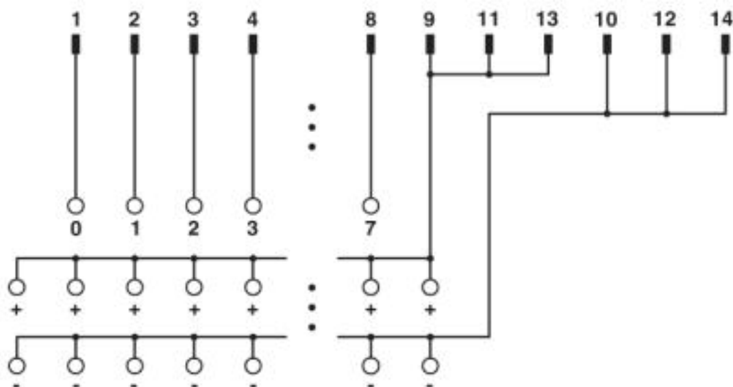
Schema di collegamento UM 45-FLK14/8IM/ZFKDS/PLC
