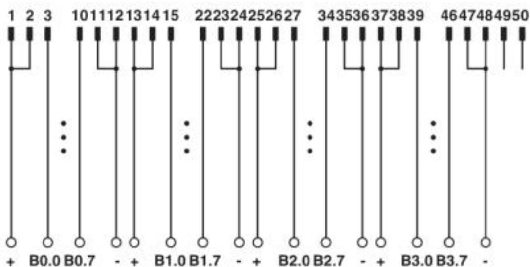
Schema di collegamento UM 45-FLK50/ZFKDS/PLC
