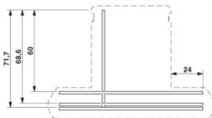
Disegno quotato
