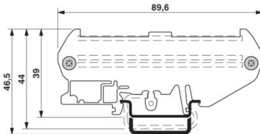
Disegno quotato
