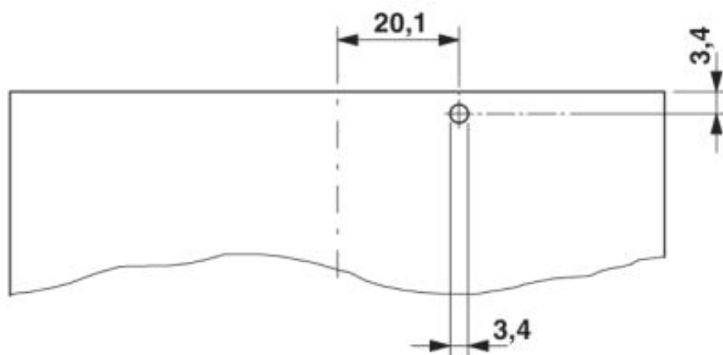
Dima di foratura
