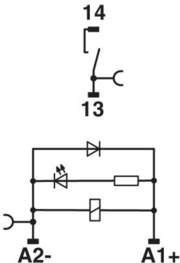
Schema di collegamento
