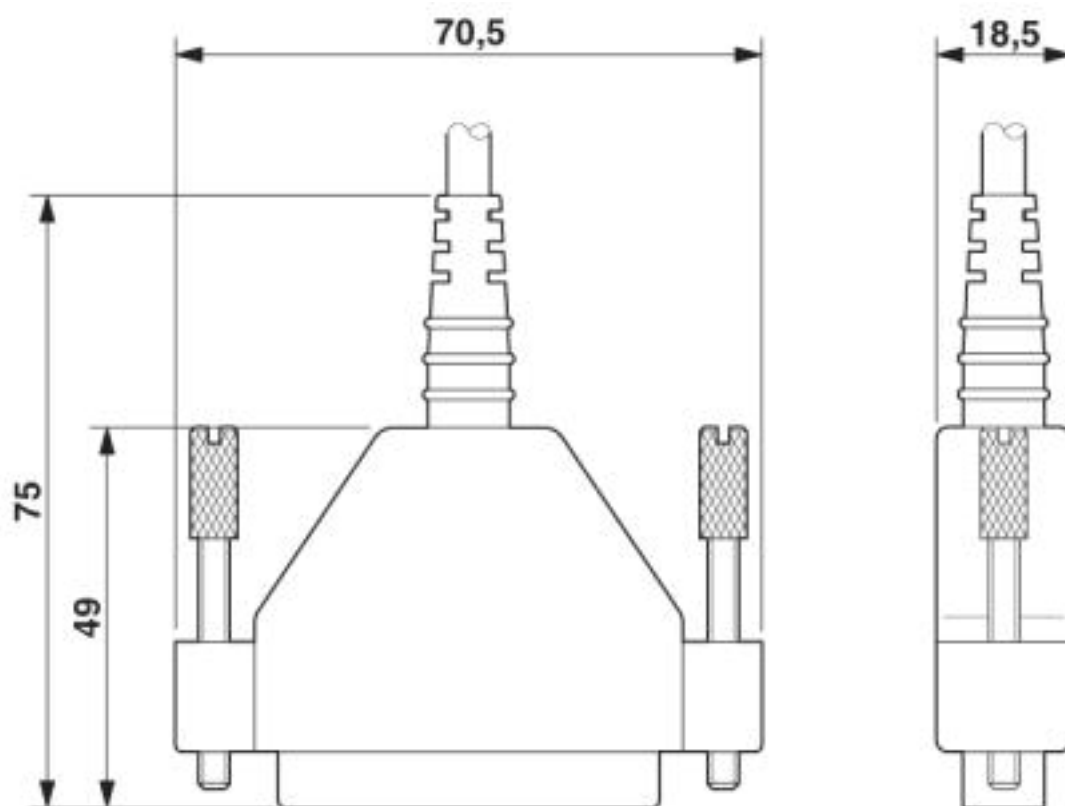
Disegno quotato
