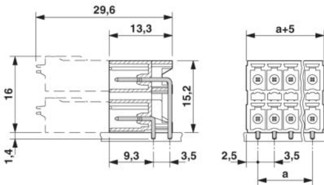
Disegno quotato
