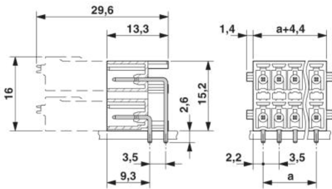
Disegno quotato
