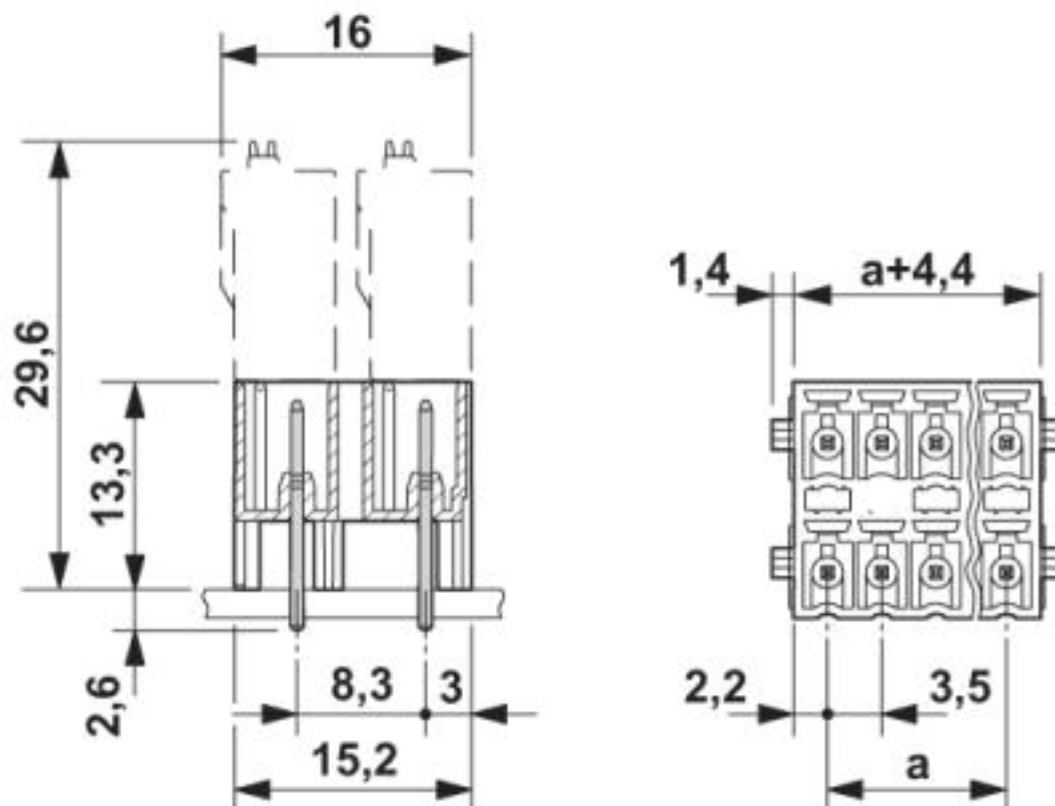
Disegno quotato
