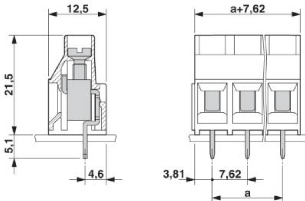
Disegno quotato
