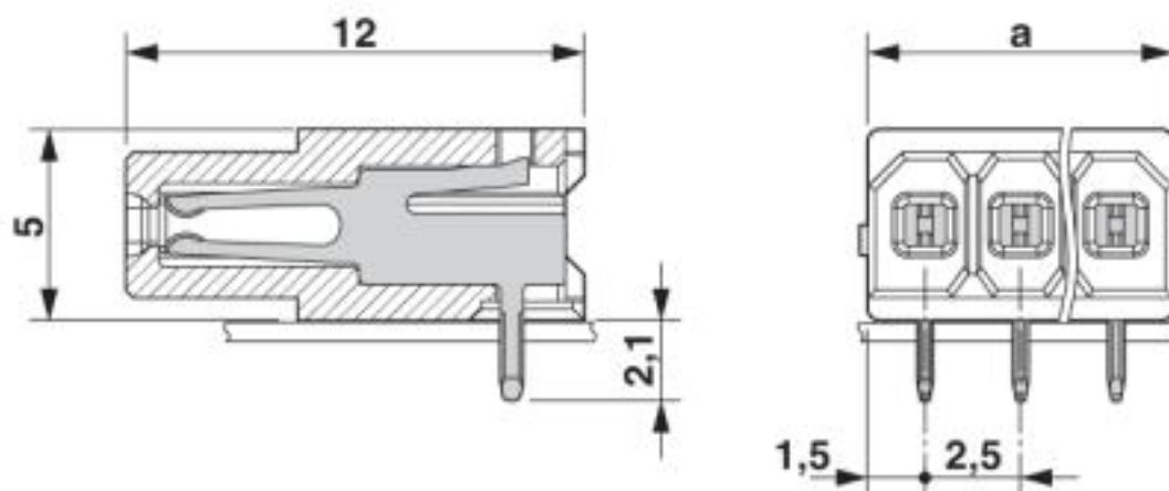
Disegno quotato
