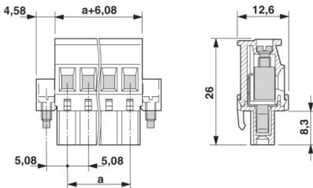
Disegno quotato
