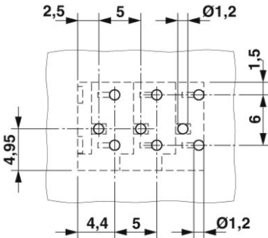
Dima di foratura
