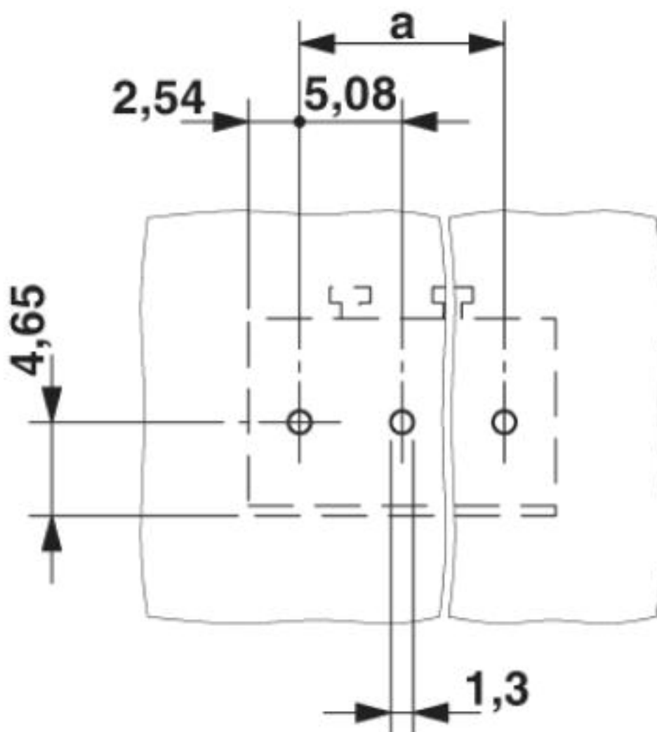
Dima di foratura
