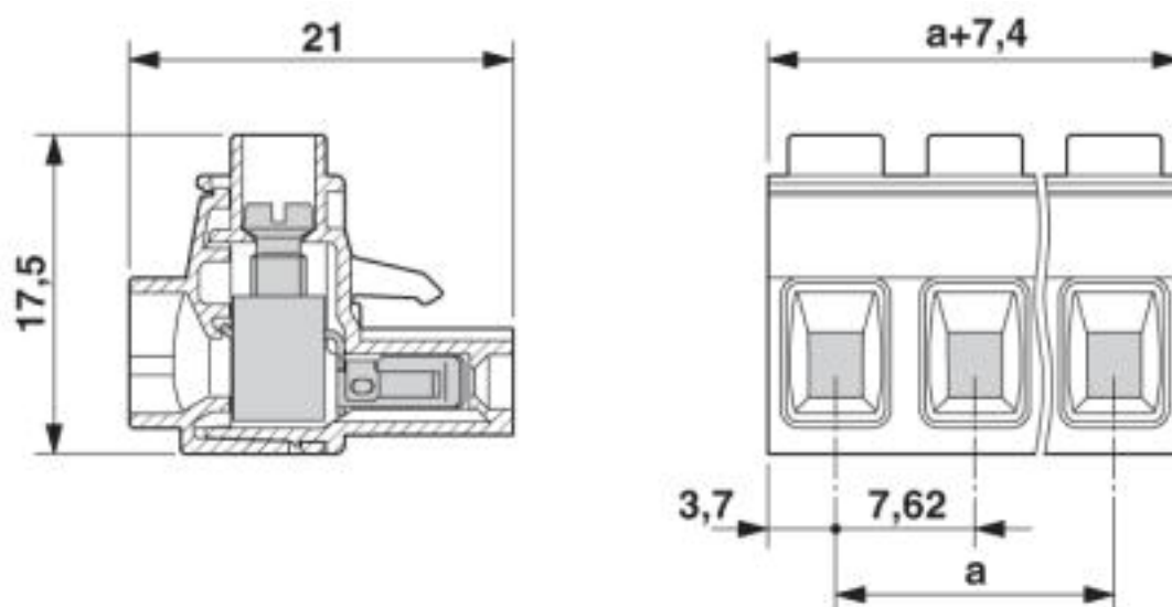
Disegno quotato
