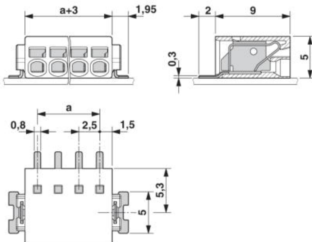
Disegno quotato
