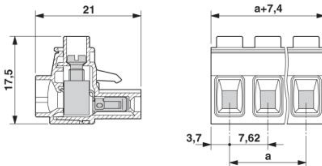
Disegno quotato
