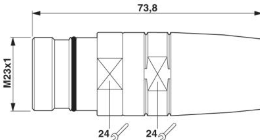
Disegno quotato
